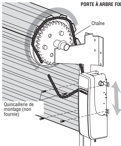
PORTE À ARBRE FIXE
