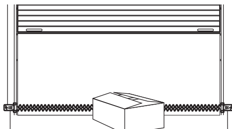
Détecteur inverseur de sécurité
