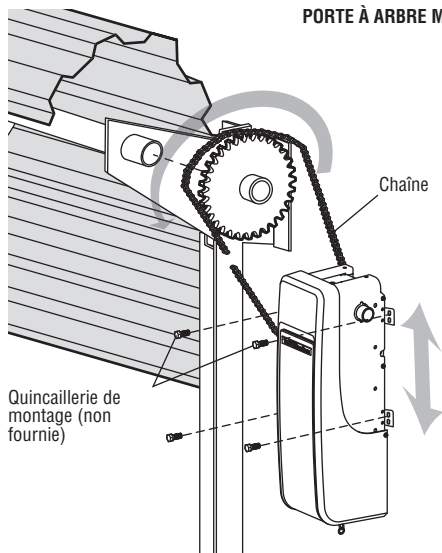
PORTE À ARBRE MOBILE
